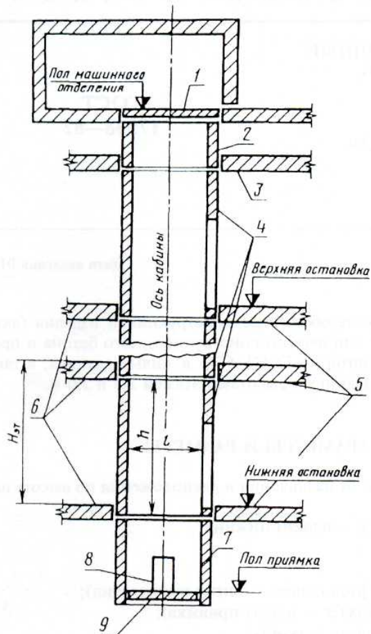
Схема шахты лифта
